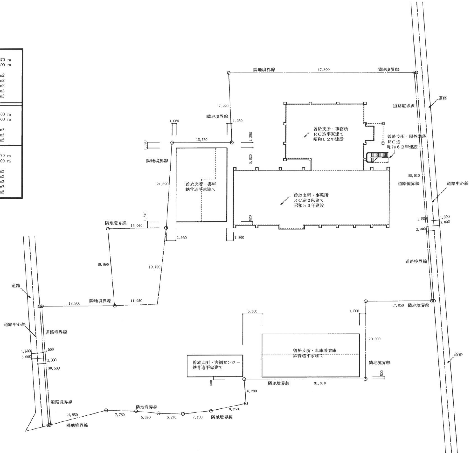
建 物 配 置 図 S = 1 / 400
